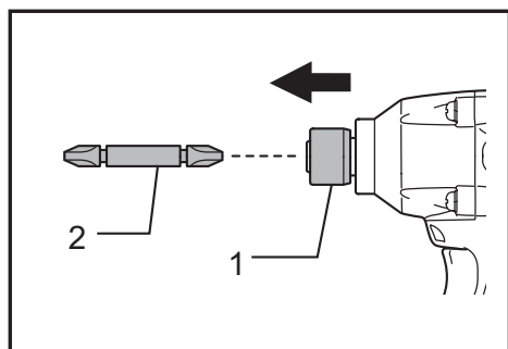
► 1. Sleeve 2. Bit
